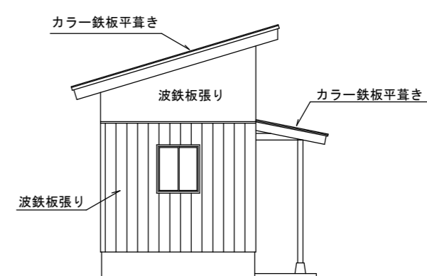
西立面図
