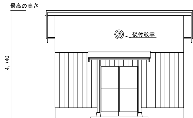
南立面図
