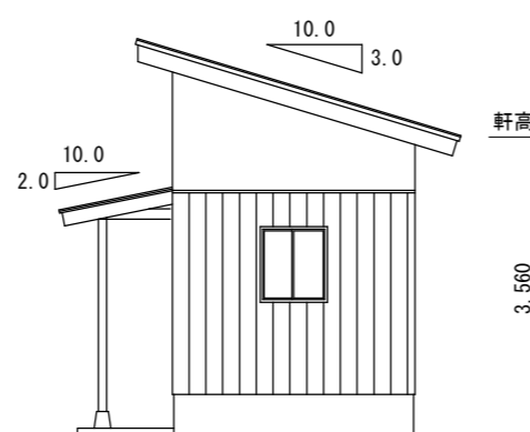
東立面図
