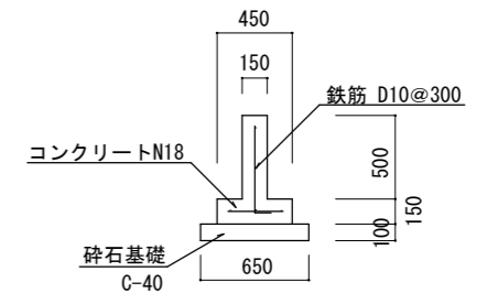
基礎断面図
