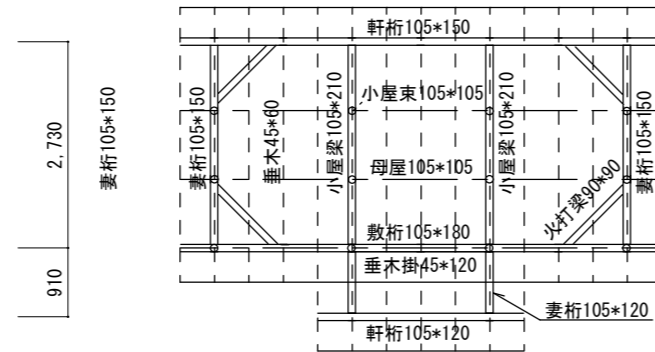
小屋伏図
