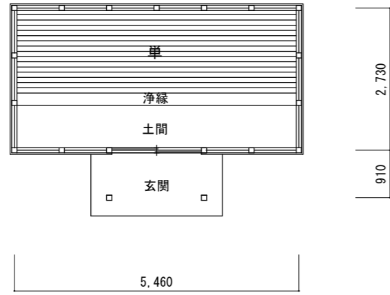
参禅堂平面图
